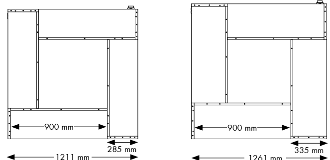
Achsmaß 900
