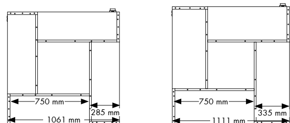
Achsmaß 750
